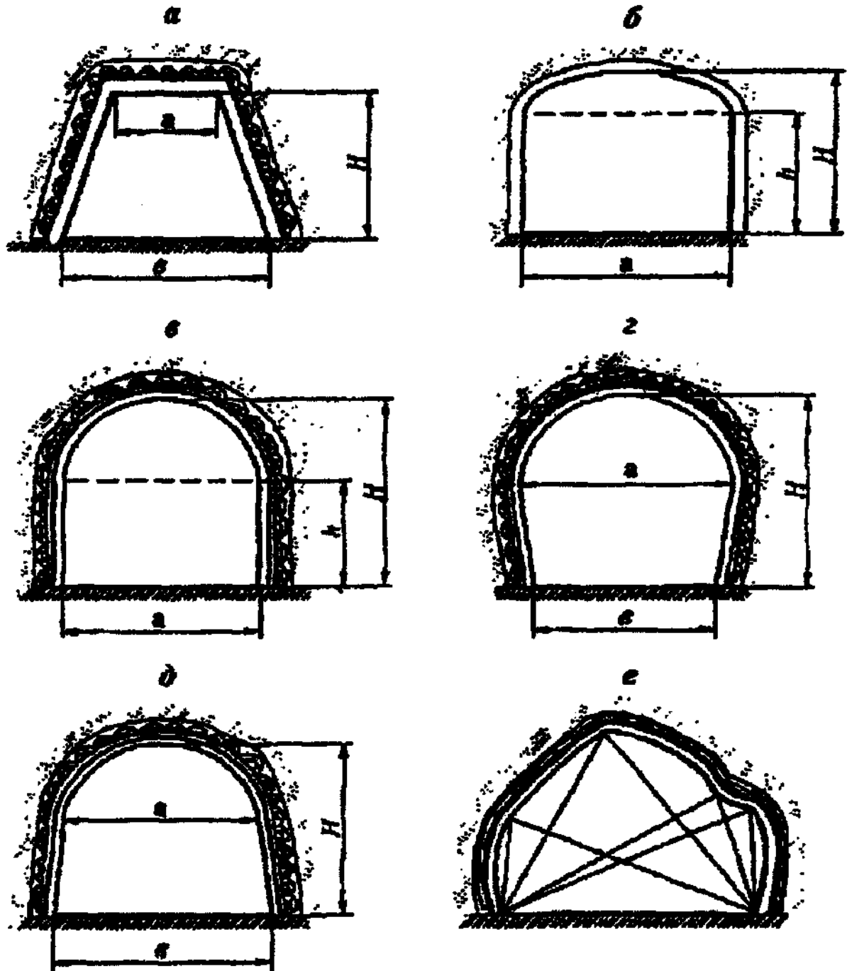
Рис. 2. Поперечные сечения горных выработок:
