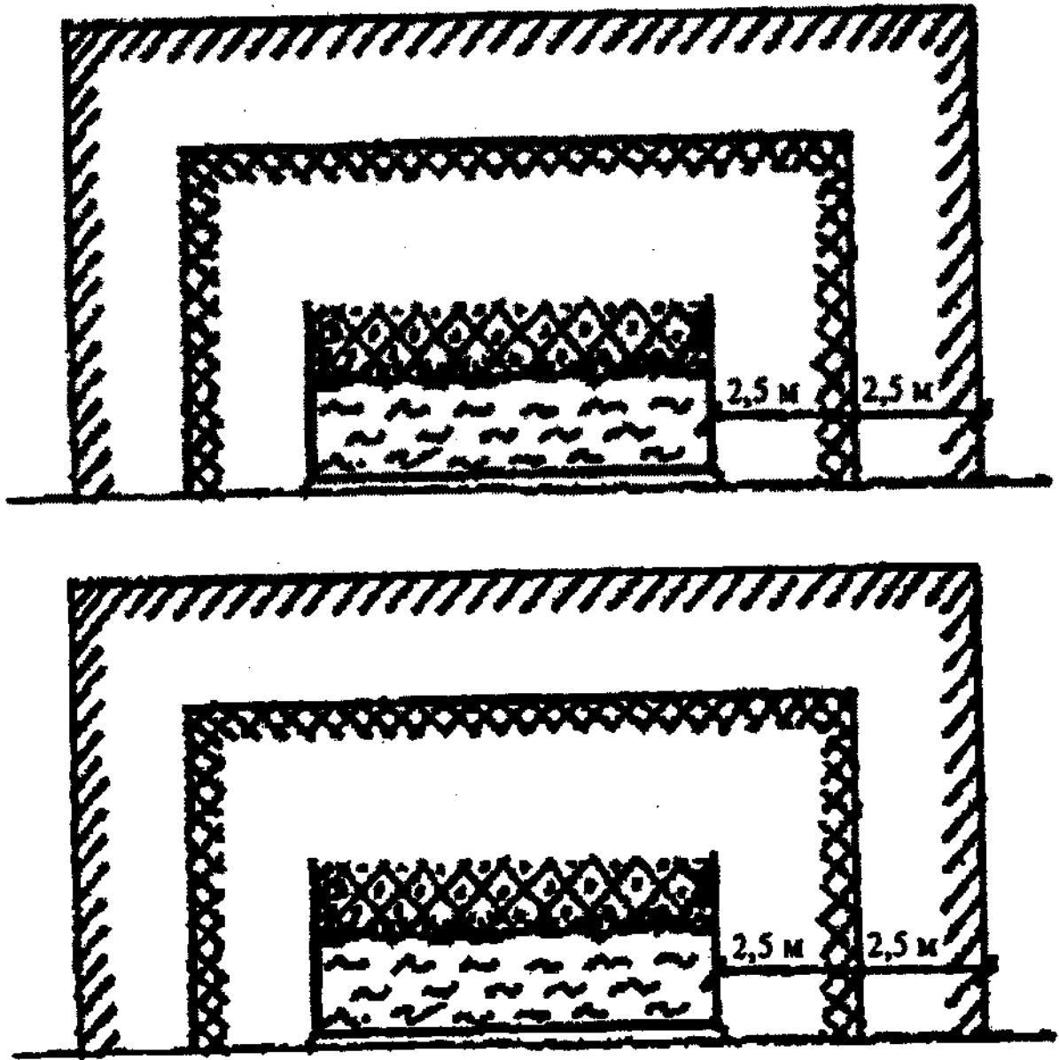
Рис. 4. Открытые пространства вокруг открытых емкостей, аппаратов, устройств
