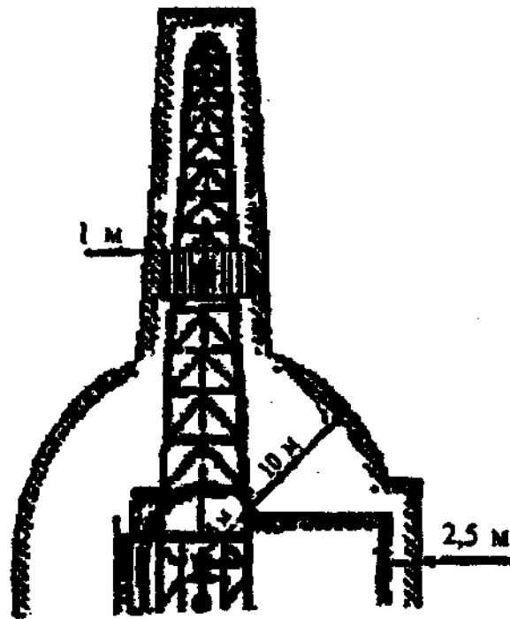
Рис. 1. Открытые емкости, аппараты, устройства в помещении
