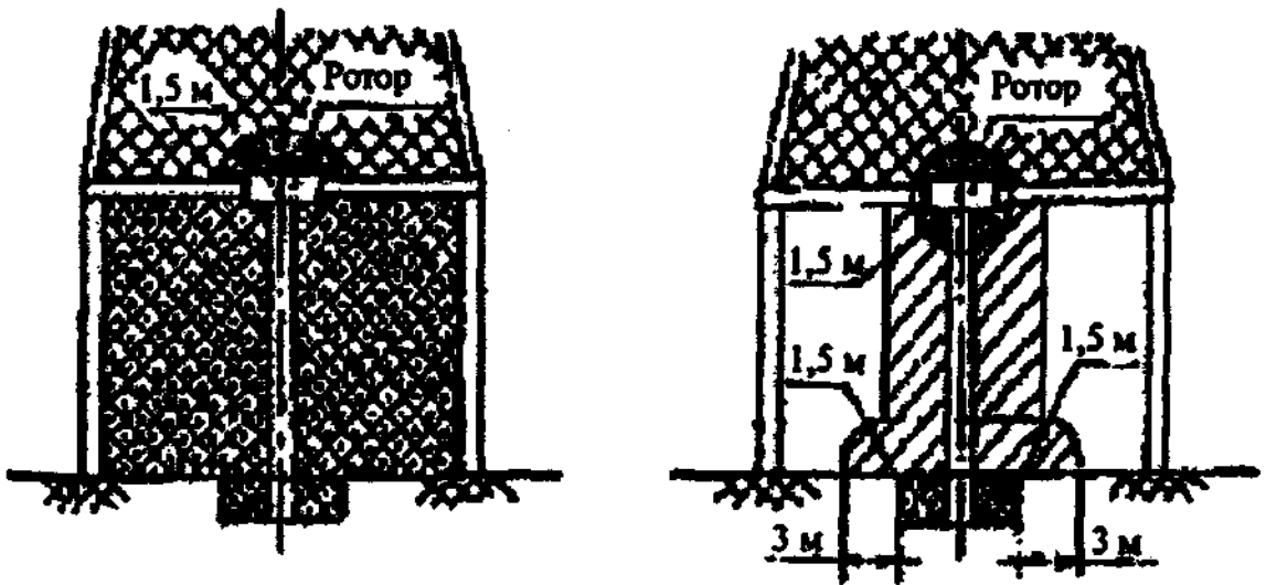
Огражденное подроторное пространство
