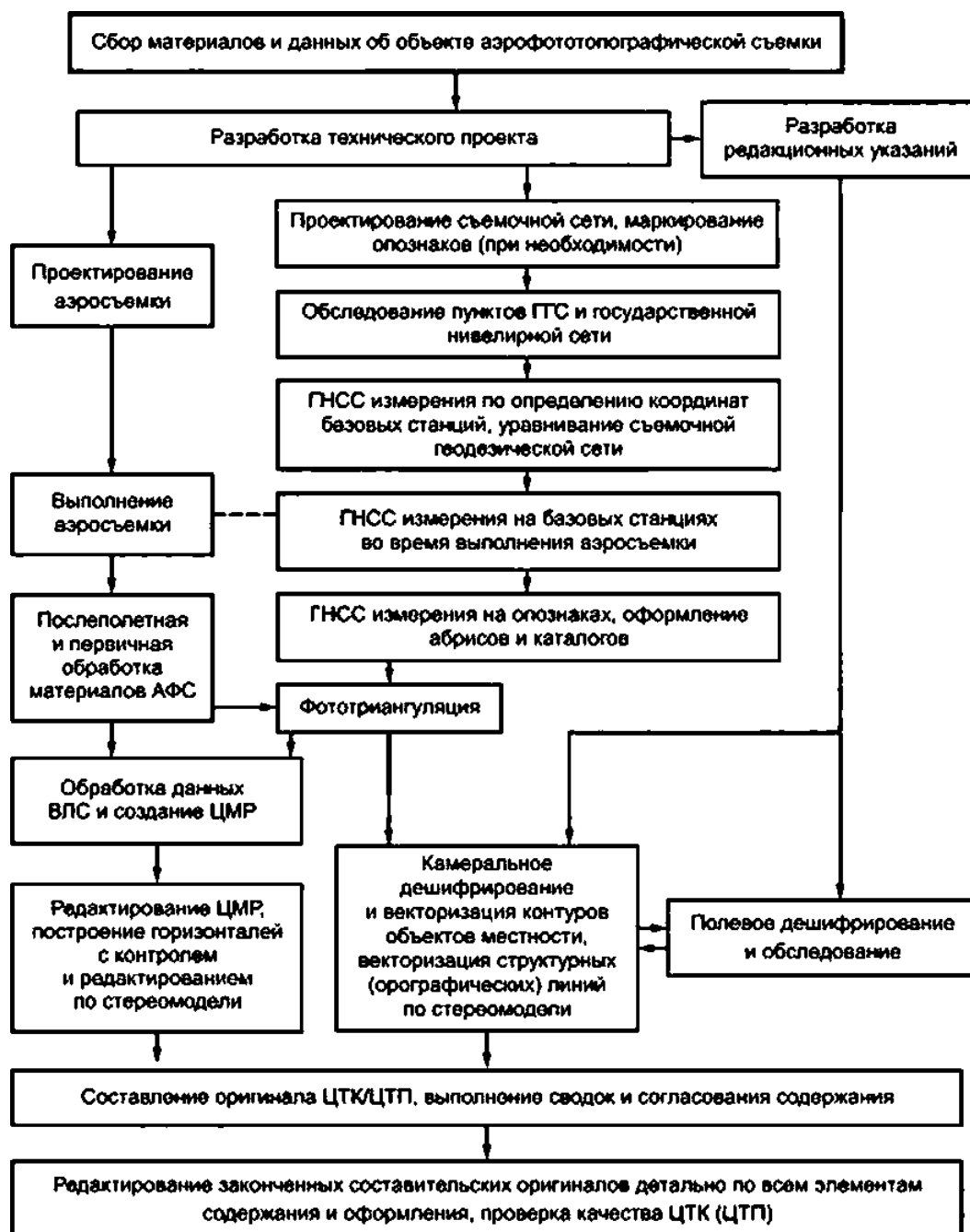
Рисунок А2 — Технологическая схема комбинированной стереотопографической съемки
