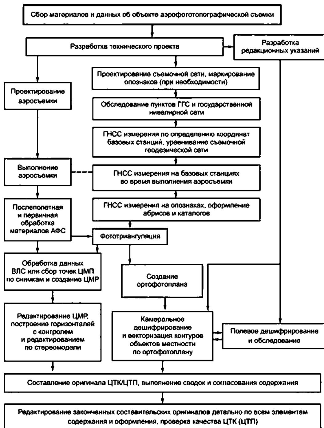
Рисунок А.3 — Технологическая схема комбинированной аэрофототопографической съемки
