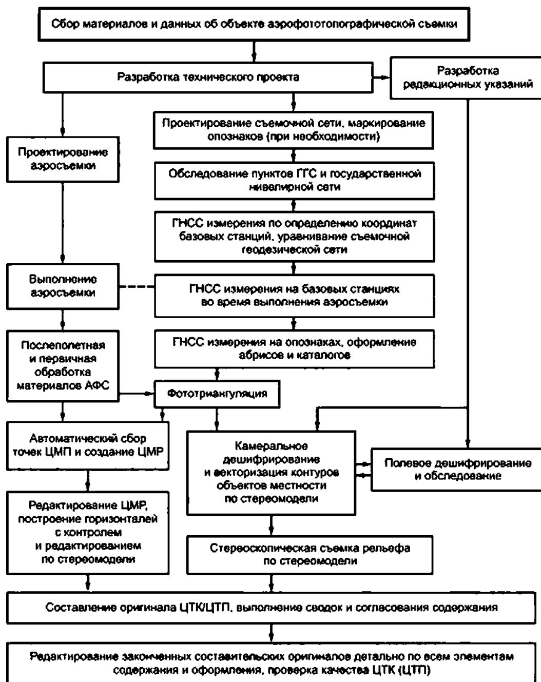
Рисунок А. 1 — Технологическая схема стереотопографической съемки
