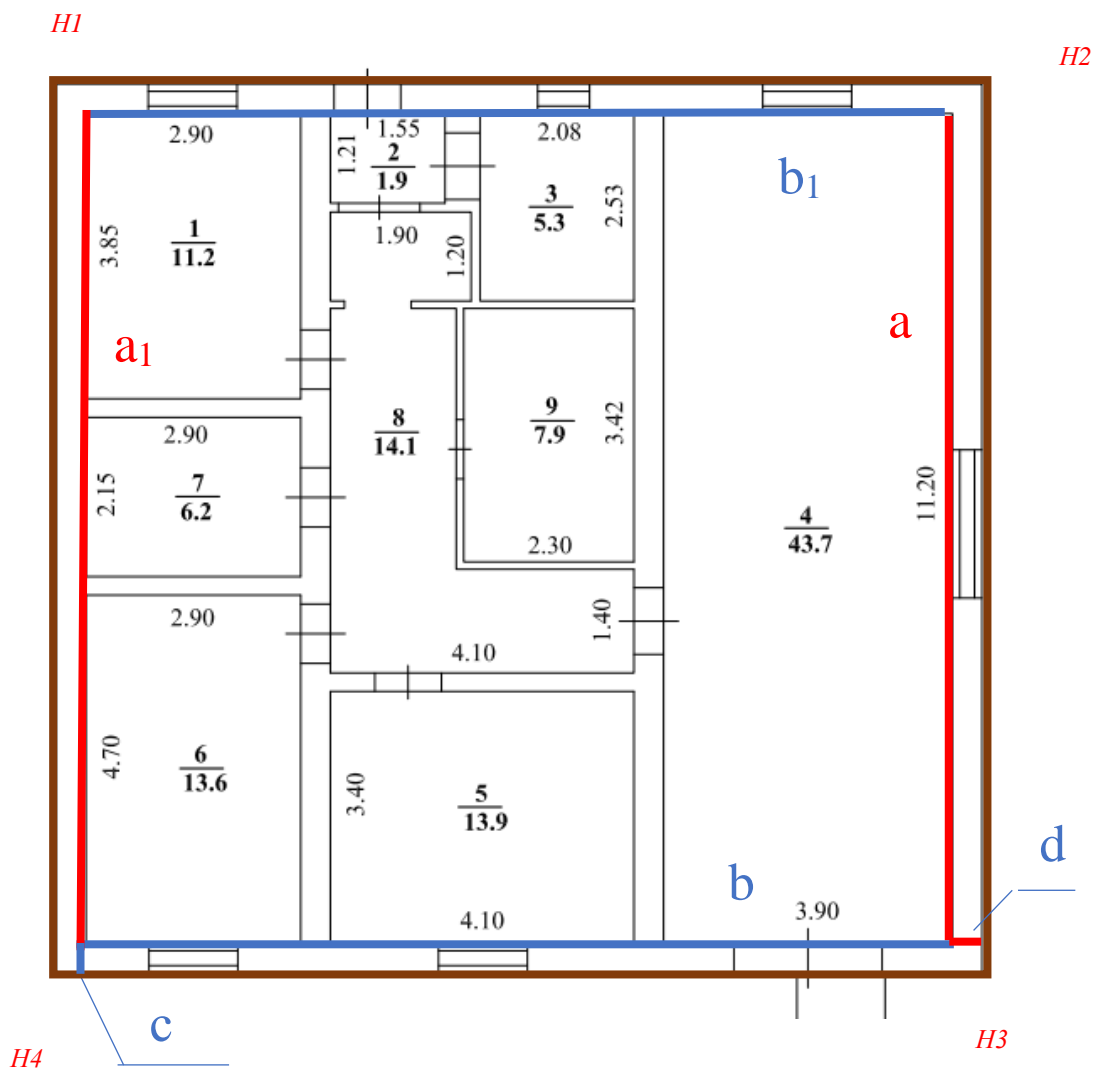
Рис. 14. Линейные измерения для расчета СКП площади здания
